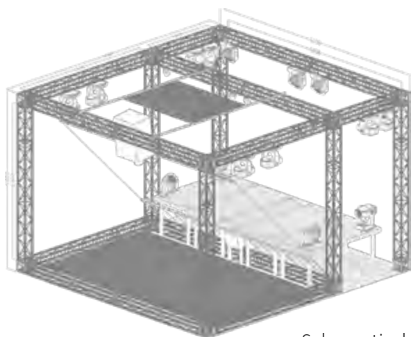
Schematischer Aufbau
