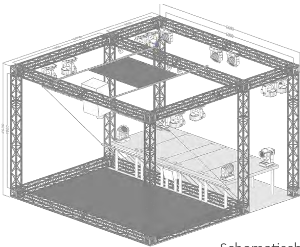
Schematischer Aufbau
